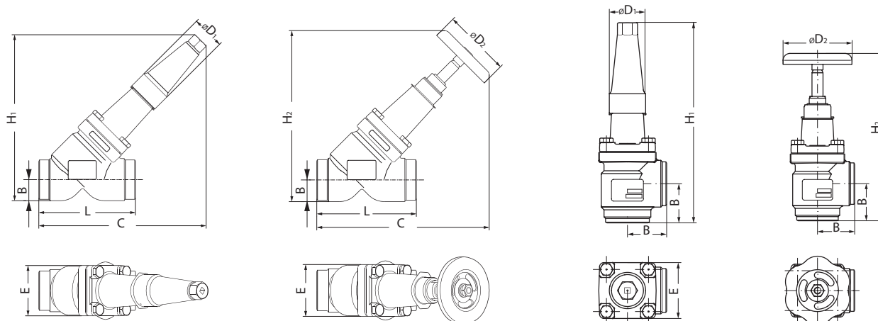
Прямые запорные клапаны SCA XXX STR
